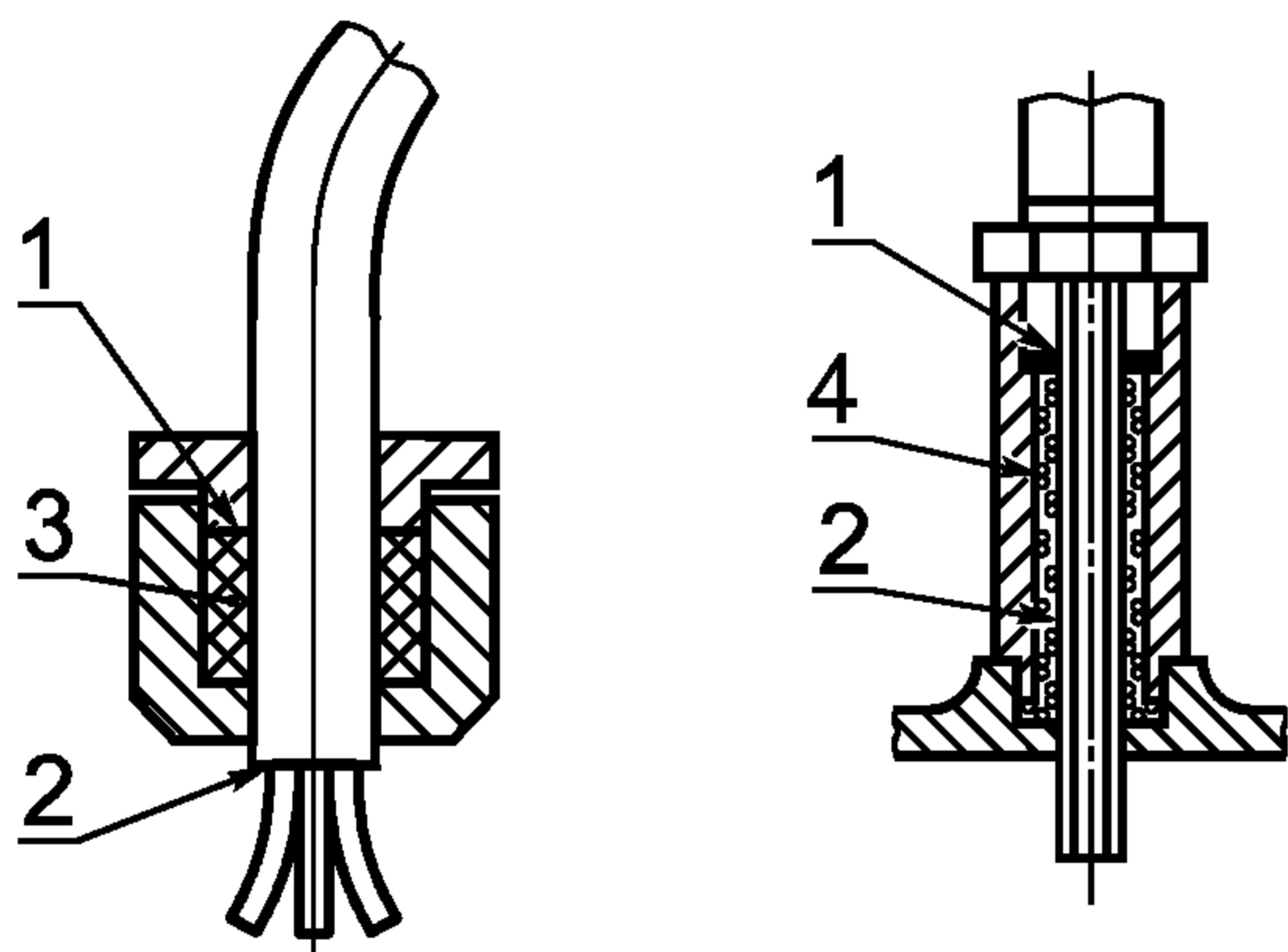
а) Кабельный ввод
