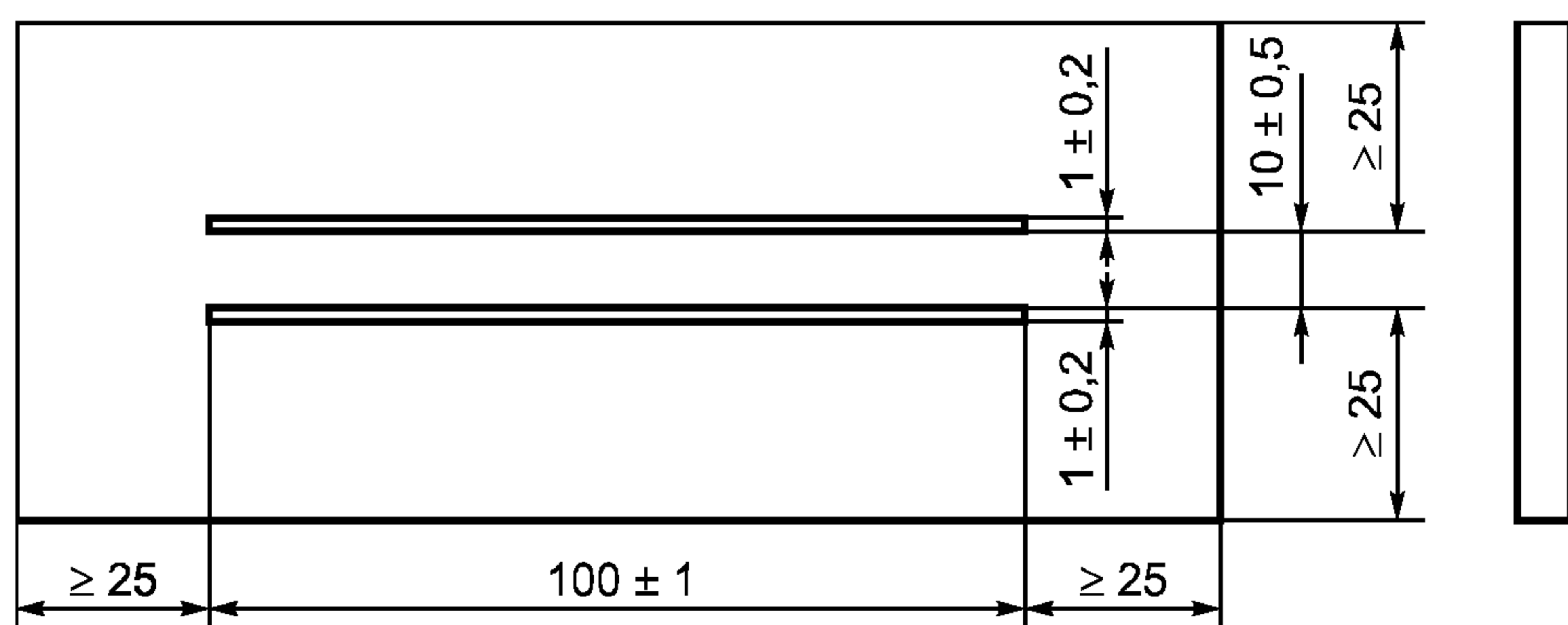
Рисунок 4 — Испытательный образец с электродами из проводящей краски
